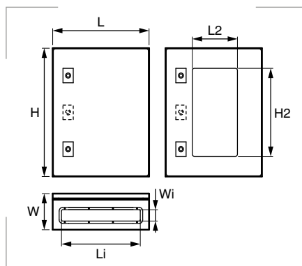
PUERTA TRANSPARENTE
